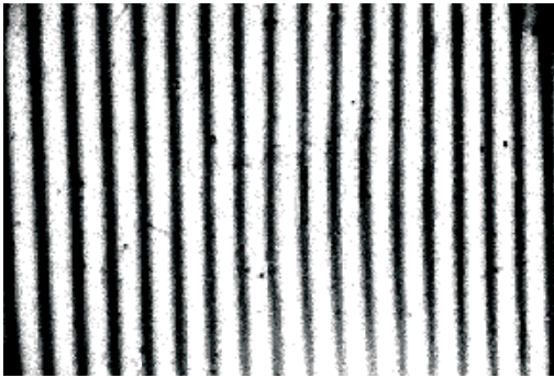
Рис. 4 Интерферограмма поверхности S1.
