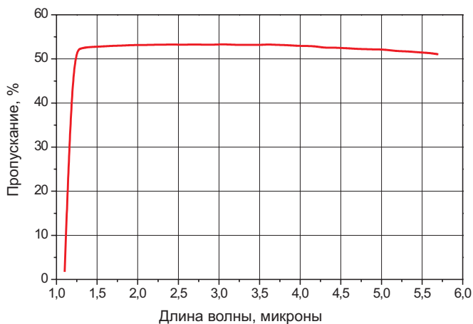
Рис. 1 Пропускание кремниевого контрольного образца №219-2-7. Толщина образца 10.0 мм.
