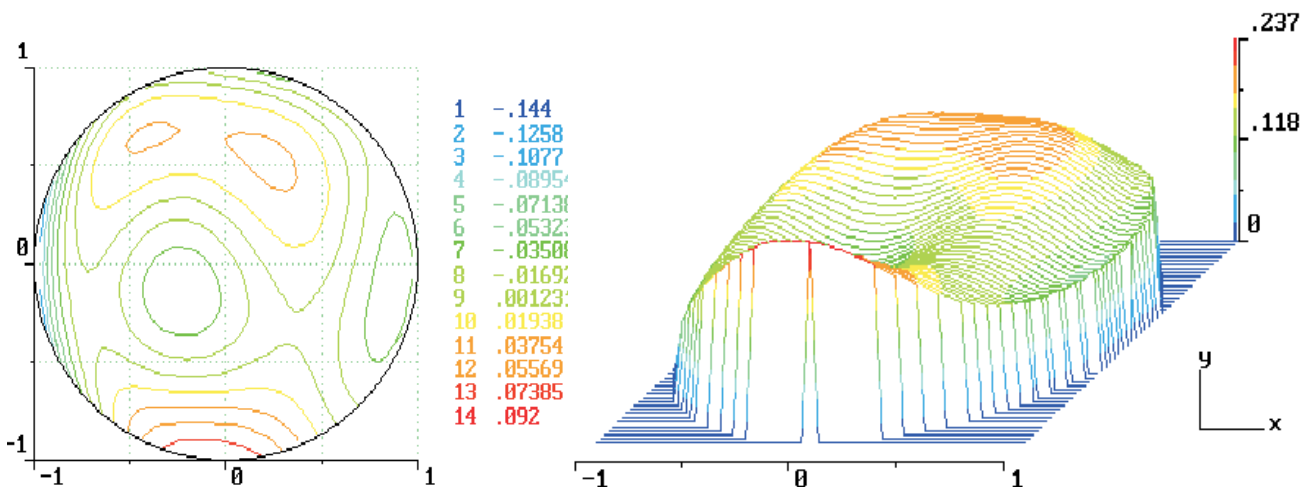
Рис. 3 Восстановленная топография искажений отраженного волнового фронта в двумерном и трёхмерном представлениях.
