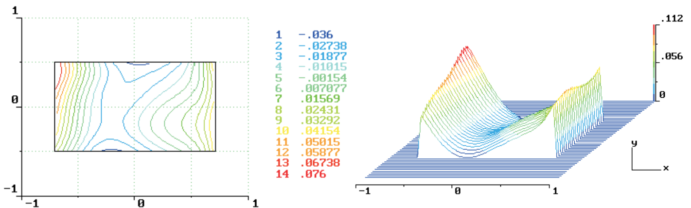
Рис. 6 Восстановленная топография искажений отраженного волнового фронта в двумерном и трёхмерном представлениях.
