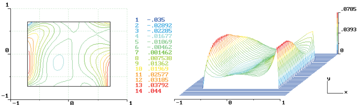
Рис. 5 Восстановленная топография искажений отраженного волнового фронта в двумерном и трёхмерном представлениях.
