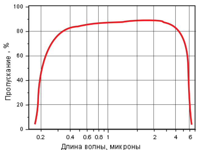
Рис. 1 Спектр пропускания сапфирового окна 2мм-толщины.
