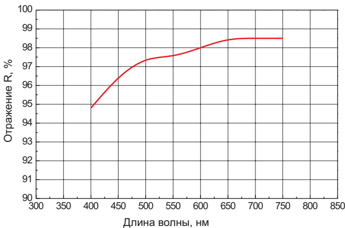
Рис. VI-4-1 Усиленное в видимой области серебряное покрытие.
