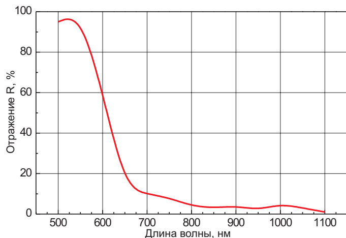
Рис. IV-1 Высокоотражающее покрытие на 532 нм и просветляющее покрытие на 1064 нм, угол падения 45°, неполяризованное излучение.
