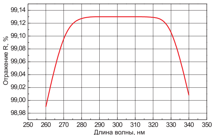
Рис. П-3-1 Высоко-отражающее покрытие на диапазон 260-340 нм, угол падения 0^\circ .
