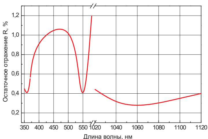
Рис I-4-3. Просветляющее покрытие для 355, 532 и 1064 нм, угол падения 0°.
