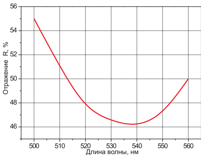
Рис. III-1-1 Светоделительное покрытие R=(50\pm 5)\% на 532 нм, угол падения 0^\circ .
