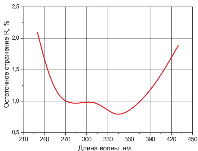
Рис. I-3-1 Просветляющее покрытие на диапазон 250-420 нм, угол падения 0°.
