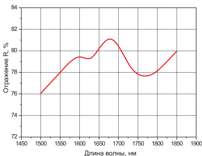
Рис. III-2-2 Светоделительное покрытие R=(80 +/-4)% на 1500-1800 нм, угол падения 0°.
