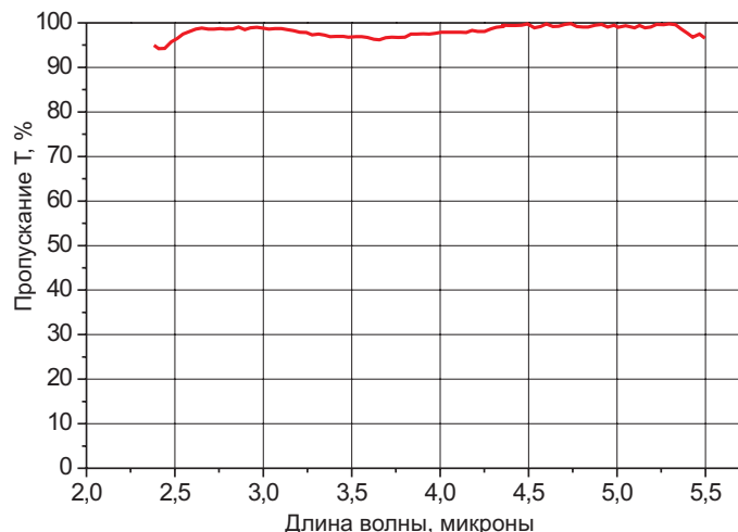
Рис. I-6-2 Просветляющее покрытие на 3-5 микрон на подложке из ZnSe, угол падения 0^\circ .
