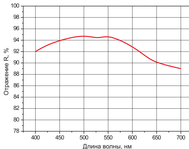
Рис. VI-2-2 Усиленное в видимой области алюминиевое покрытие.
