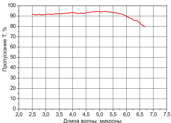
Рис. I-6-1 Просветляющее покрытие на 2-6 микрон на подложке из Si, угол падения 0^\circ .
