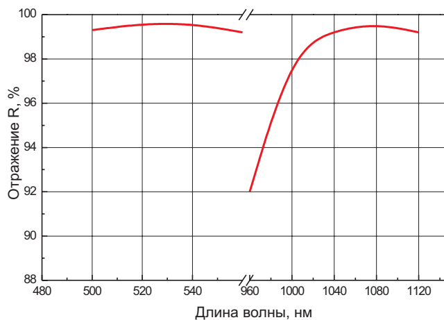
Рис. П-2-2 Зависимость отражения от длины волны для высоко-отражающего покрытия. R > 99.5\% на 532 нм и 1064 нм, угол падения 0^\circ .
