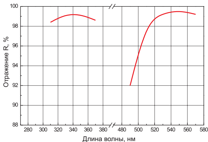
Рис. П-2-1 Зависимость отражения от длины волны для высоко-отражающего покрытия. R > 99\% на 355 нм и R > 99.5\% на 532 нм, угол падения 0^\circ .
