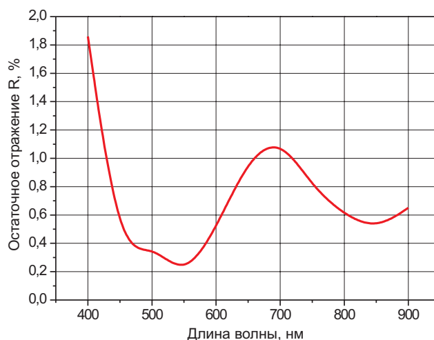
Рис. I-3-2 Просветляющее покрытие на диапазон 425-675 нм, угол падения 0°.
