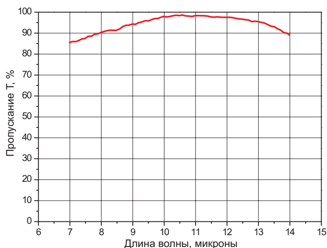
Рис. I-5-1 Просветляющее покрытие на 10.6 микрона на подложке из ZnSe, угол падения 0°.
