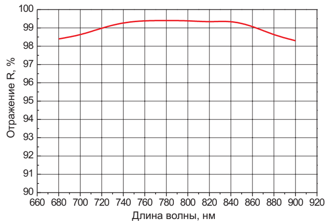
Рис. VI-4-2 Усиленное в ближней ИК области серебряное покрытие.
