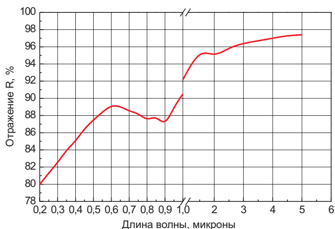
Рис. VI-1 Алюминиевое покрытие с защитой для диапазона 0.2-10 микрон.
