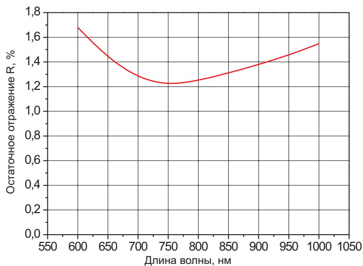
Рис. I-1 Однослойное просветляющее покрытие MgF_2 на диапазон длин волн 600-1000нм, угол падения 0^\circ .
