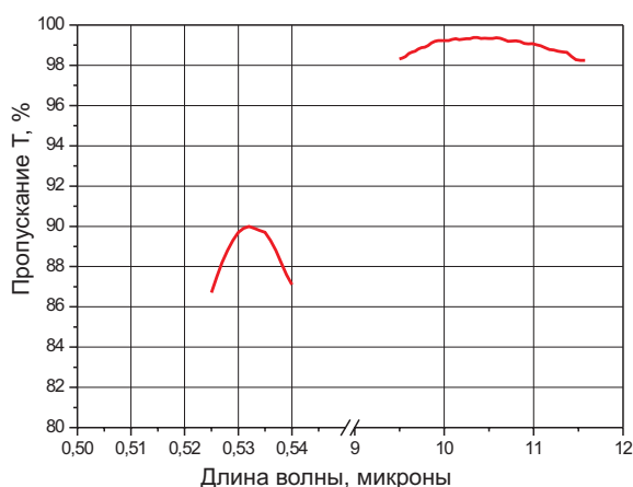
Рис. I-7-1 Просветляющее покрытие на 532 нм и 10,6микрона на ZnSe, угол падения 0^\circ .
