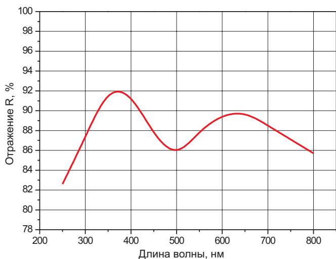
Рис. VI-2-1 Усиленное в УФ алюминиевое покрытие.
