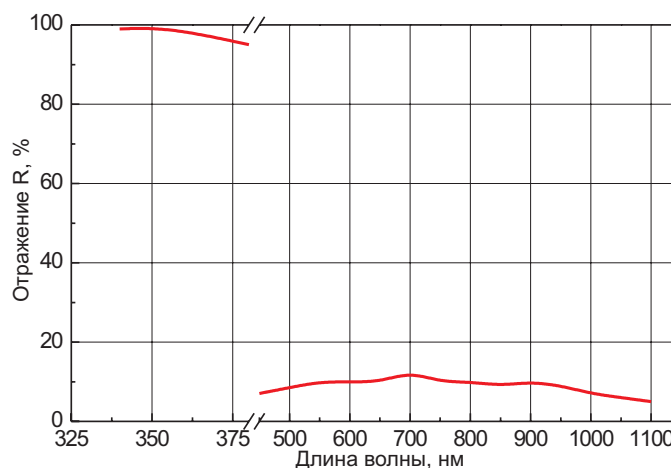
Рис. IV-2 Высокоотражающее покрытие на 355 нм и просветляющее просветление на 532 и 1064 нм, угол падения 0°.
