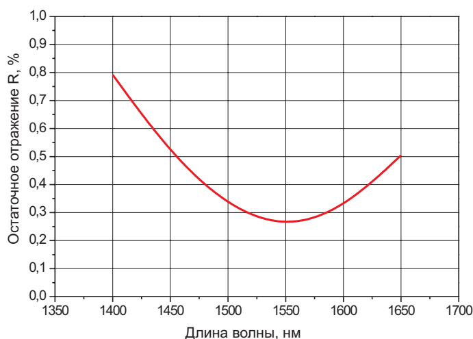
Рис. I-2-2 Просветляющее покрытие на 1550 нм, угол падения 0^\circ .
