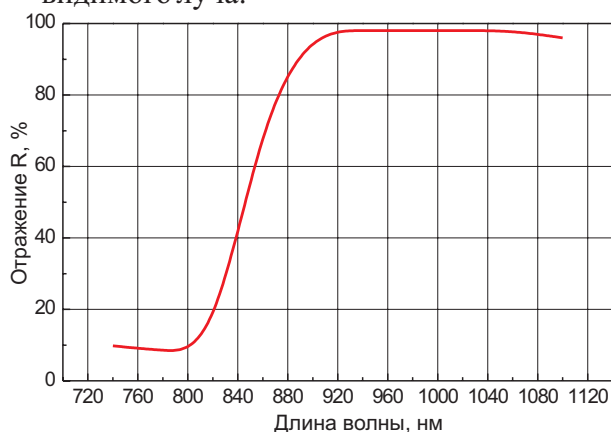
Рис. V-1 "Горячее" зеркало на диапазон 740-820/900-1100 нм, угол падения 0°.
