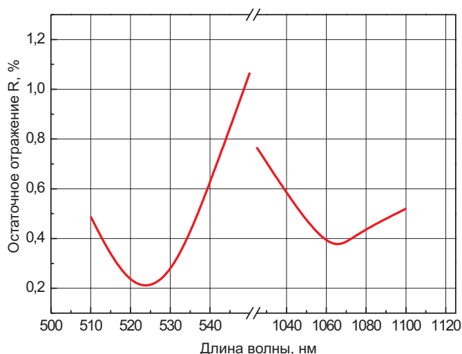
Рис. I-4-2 Просветляющее покрытие для 532 и 1064 нм, угол падения 0°.
