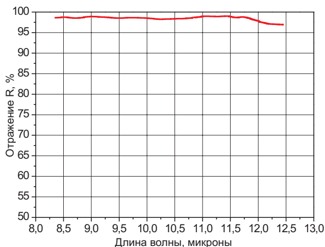
Рис. VII-7-2 Усиленное золотое покрытие на 10.6 микрона.
