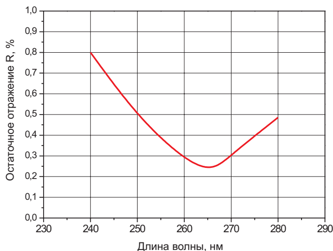
Рис. I-2-1 Просветляющее покрытие на 266 нм, угол падения 0^\circ .
