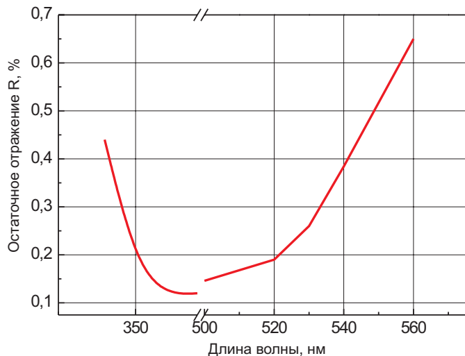
Рис. I-4-1 Просветляющее покрытие для 355 и 532 нм, угол падения 0°.
