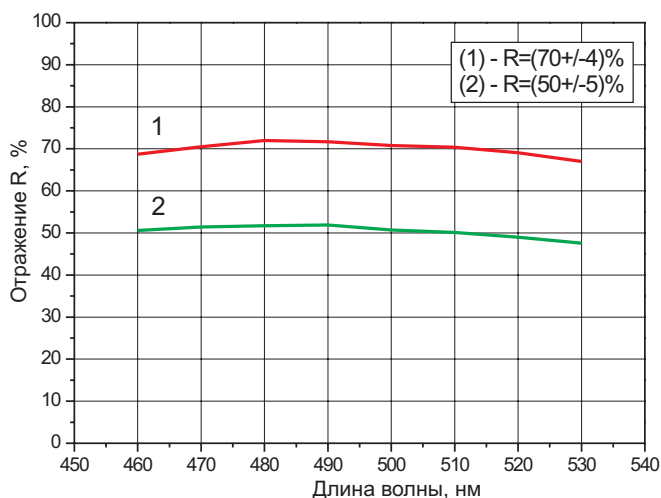
Рис. III-2-1 Светоделительное покрытие на 470-520 нм для S- и P-поляризации, угол падения 45°.
