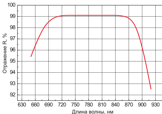
Рис. П-3-2 Высоко-отражающее покрытие на диапазон 700-900 нм, угол падения 0^\circ .
