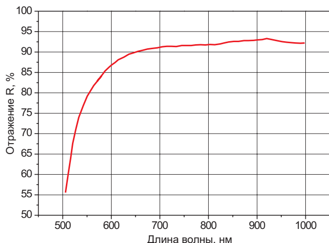
Рис. VII-7-1 Усиленное золотое покрытие на 532 нм.
